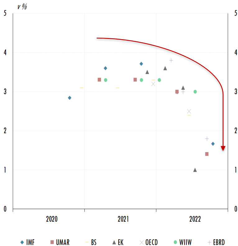
Napovedi realne rasti BDP za Slovenijo za 2023
